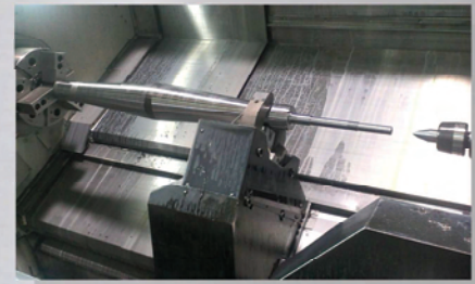
Torno de control numérico OKUMA LB4000 EX Capacidad de trabajo: Volteo de 480 y 2000 de longitud
